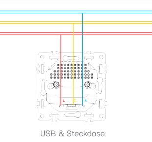
Steckdose
